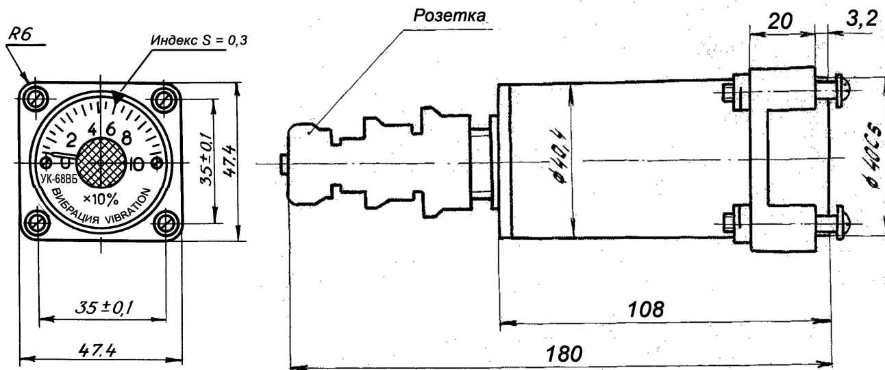
Указатель УК-68ВБ. Габаритные размеры
