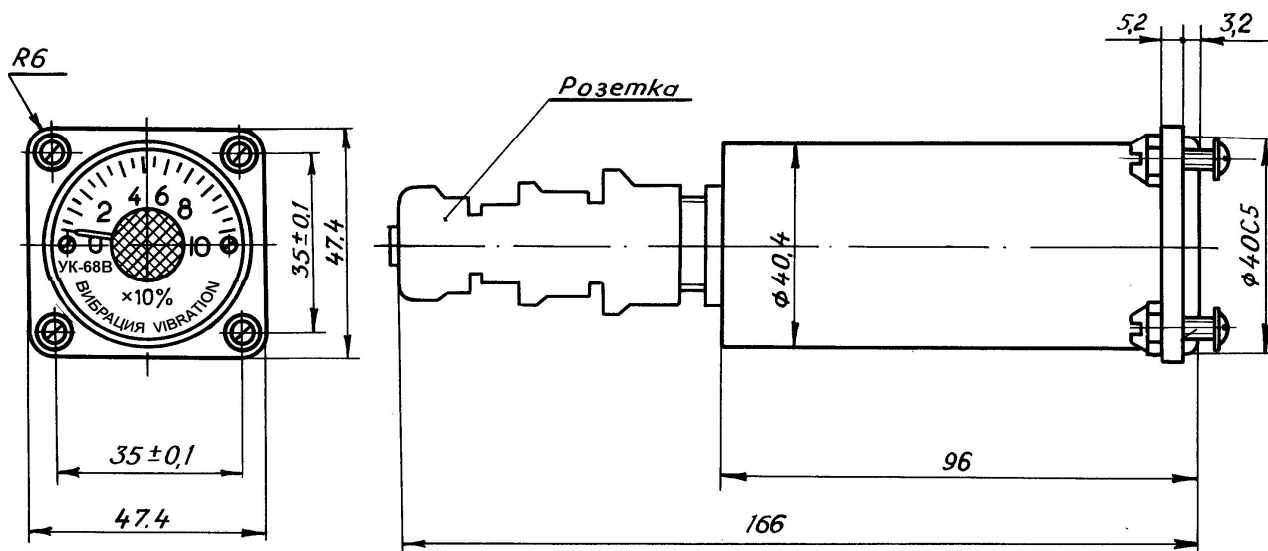
Указатель УК-68В. Габаритные размеры
